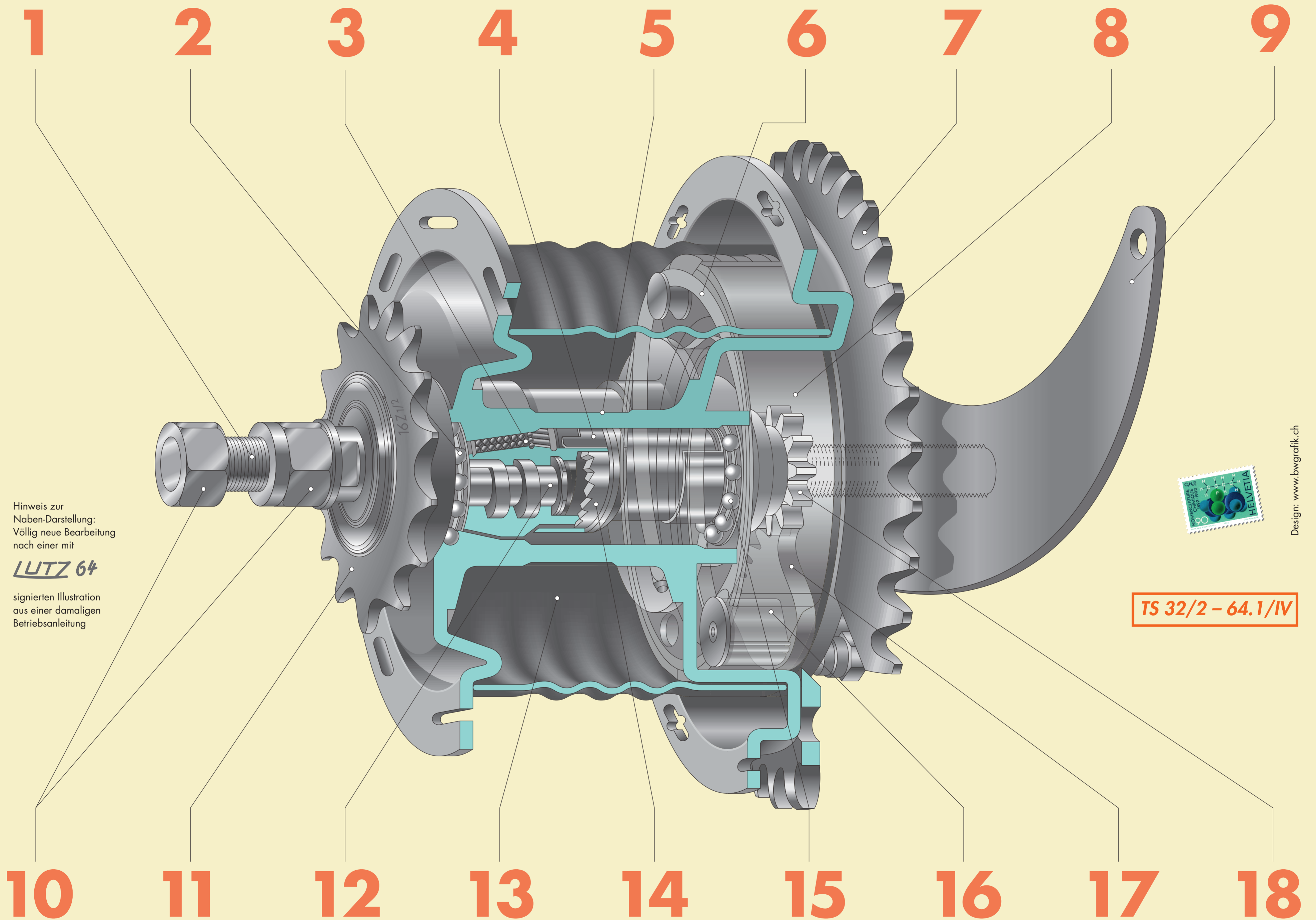
Tafel III: Hinterradnabe (Schnittbild)
